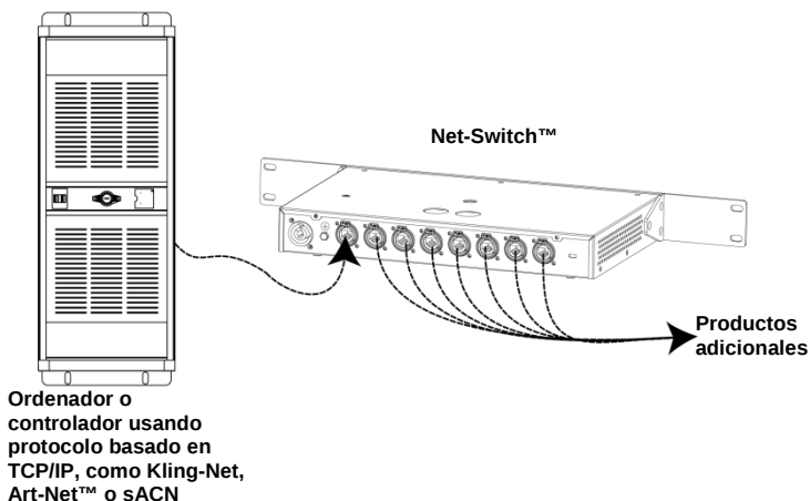
Diagrama de conexiones Ethernet
