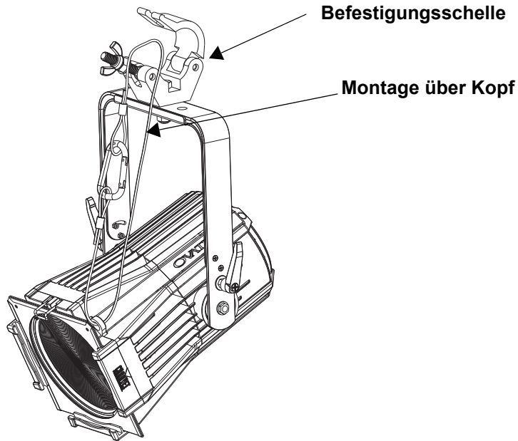
Montageansicht
