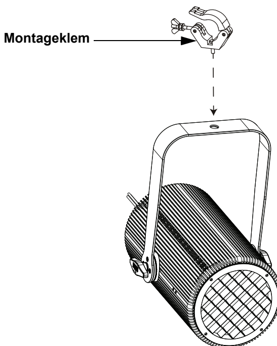
Montage boven het hoofd
