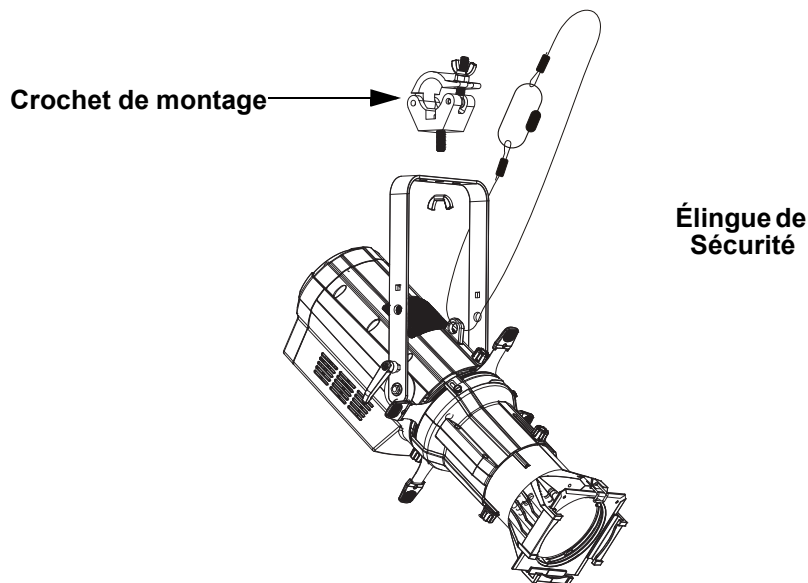
Montage en hauteur
